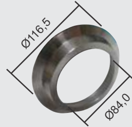
FLANGE AÇO Ø INT. 84,00mm X Ø EXT. 116,50
