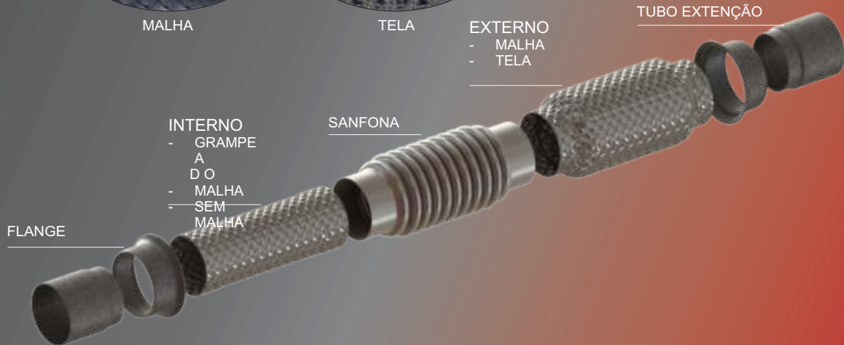
TUBO EXTENÇÃO
