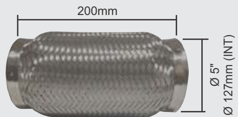
FLEXIVEL MALHA Ø INT. 5" (127mm) X 200mm S/ TUBO INT. GRAMPEADO
