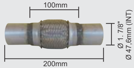
FLEXIVEL MALHA DUPLA Ø INT. 1. 7/8" (47,6mm) X 100mm X 200mm
