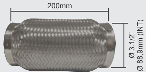
FLEXIVEL MALHA Ø INT. 3.1/2" (88,9mm) X 200mm S/ TUBO INT. GRAMPEADO
